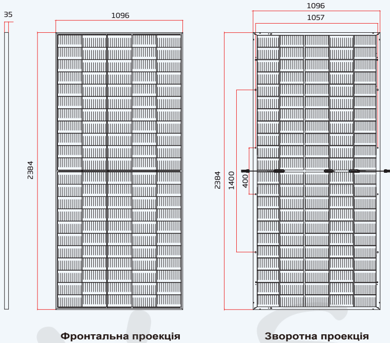
Фронтальна проекція
